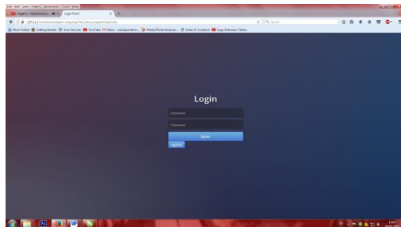
Gambar 4.9 Tampilan Login
