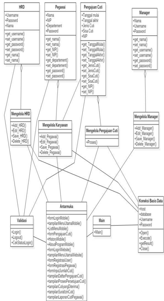
Gambar 3.4 Diagram Kelas
